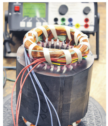
Mit Kupferdraht bewickeltes Statorpaket eines Elektromotors.
